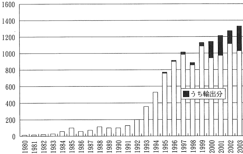
図2 中国の二輪車の生産台数と輸出 (単位: 万台)
